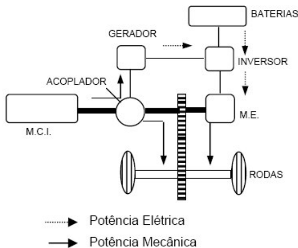
Esquema 2: Configuração Mista [15] .
