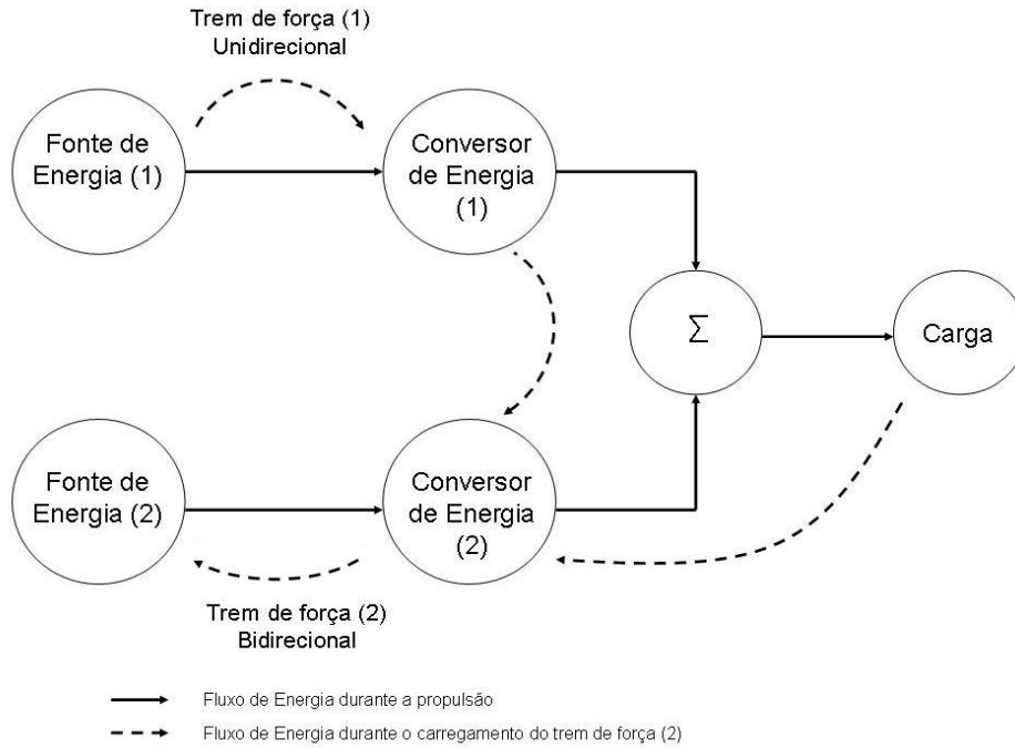
Esquema 1: Conceito de sistema de transmissão de um veículo elétrico híbrido [14] .
